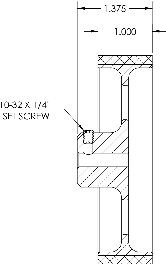
SECTION A-A
